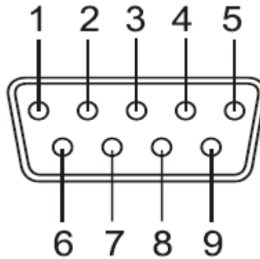
D-Sub 9 Pin
