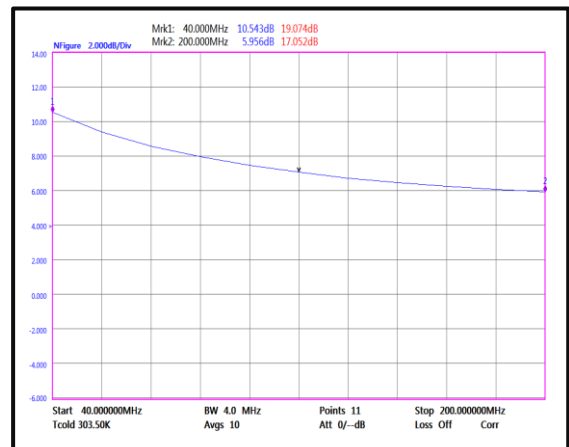
Noise Figure(0.04-0.2GHz)
