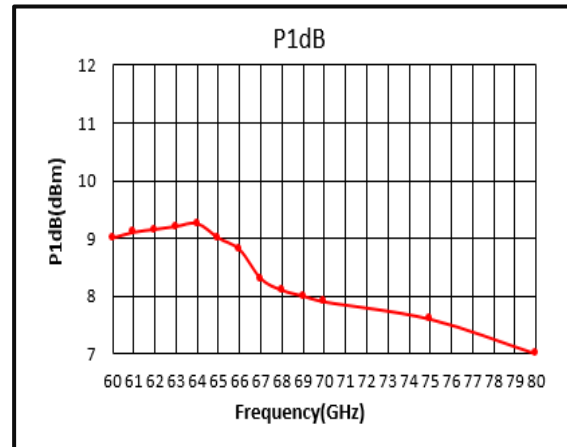
P1dB(60-80GHz)
