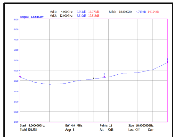
Noise Figure(4GHz-18GHz)
