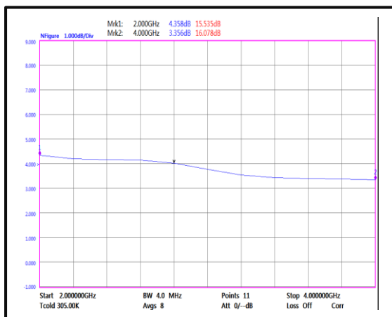
Noise Figure(2GHz-4GHz)
