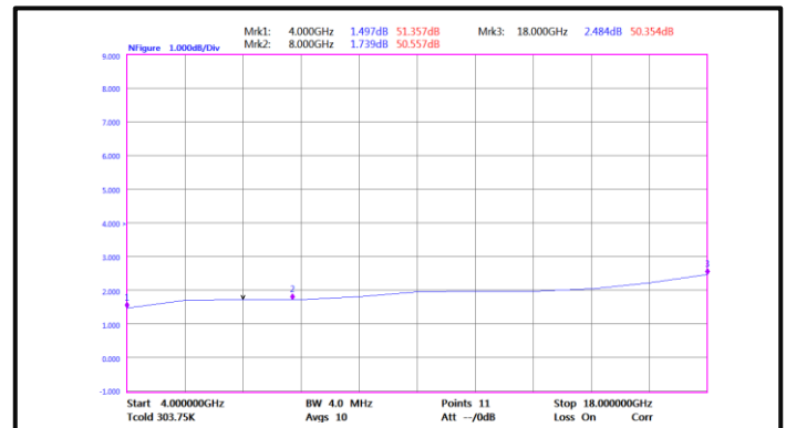
Noise Figure(4GHz-18GHz)
