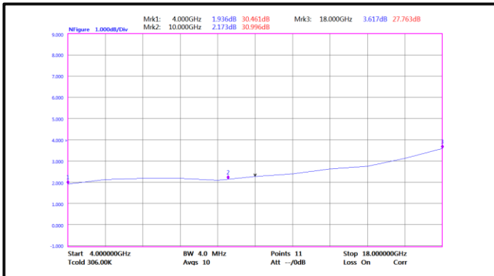
Noise Figure(4-18GHz)
