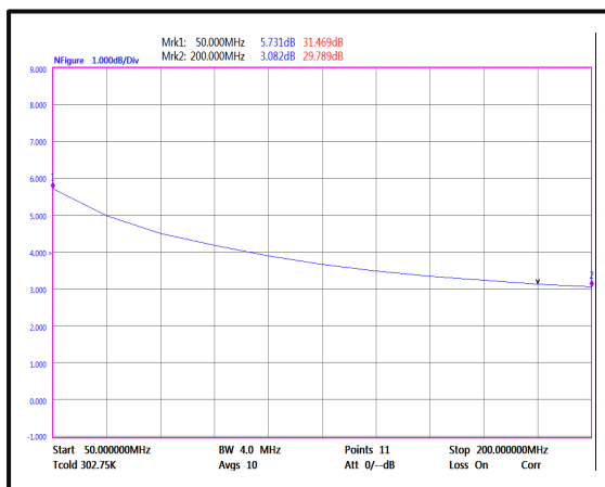
Noise Figure(50MHz-200MHz)
