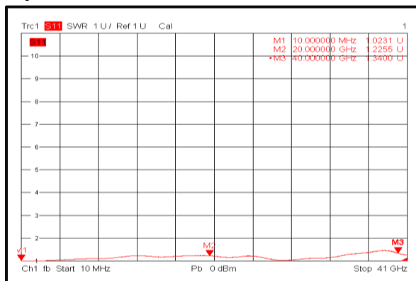
Input VSWR
