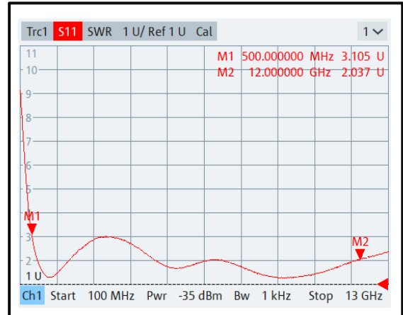
Input VSWR@+85°C
